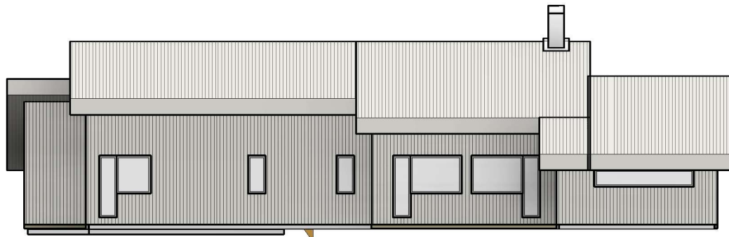
Fasade Nord 1 : 100
