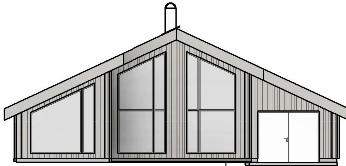
Fasade Vest 1 : 100
