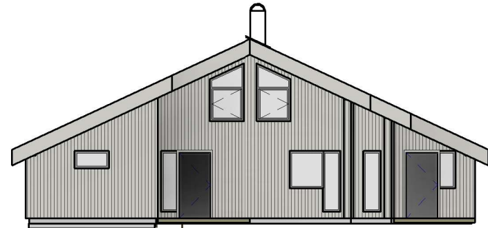
Fasade Øst 1 : 100
