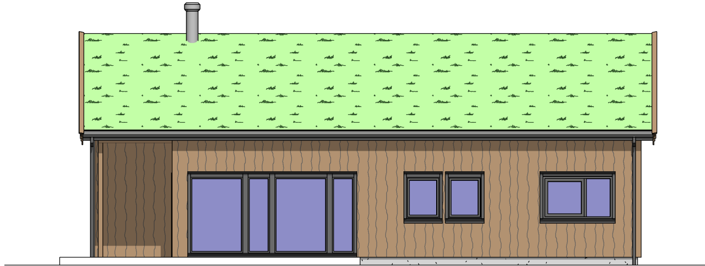
Fasade 1 1 : 100
