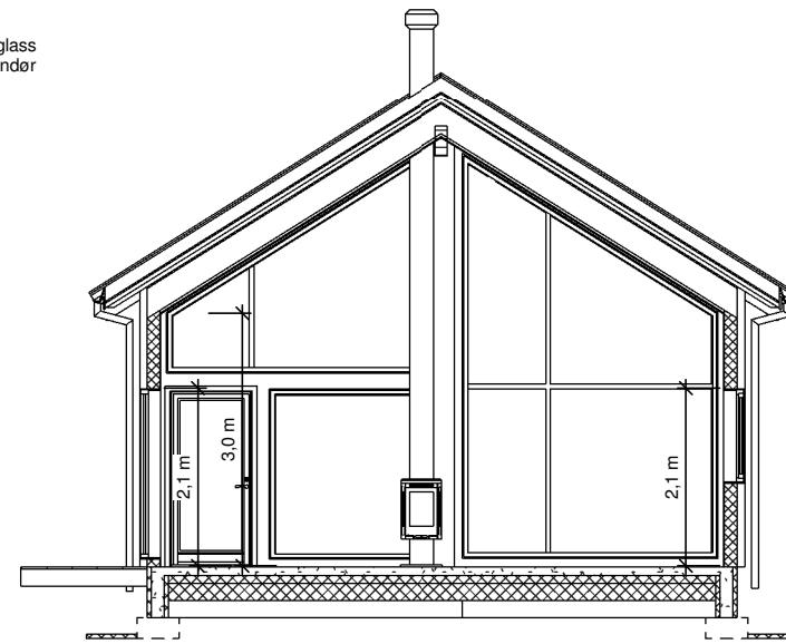
Snitt B 1 : 100
