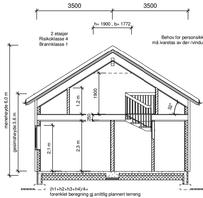
Snitt A 1 : 100
