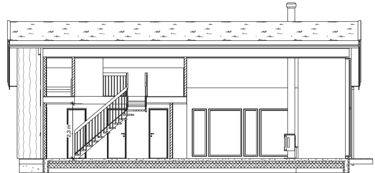
Snitt C 1 : 100
