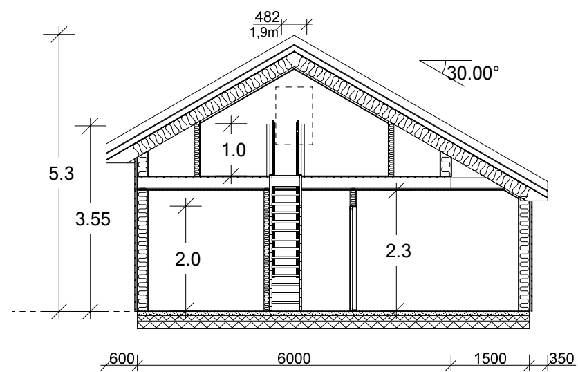
Snitt A-A
