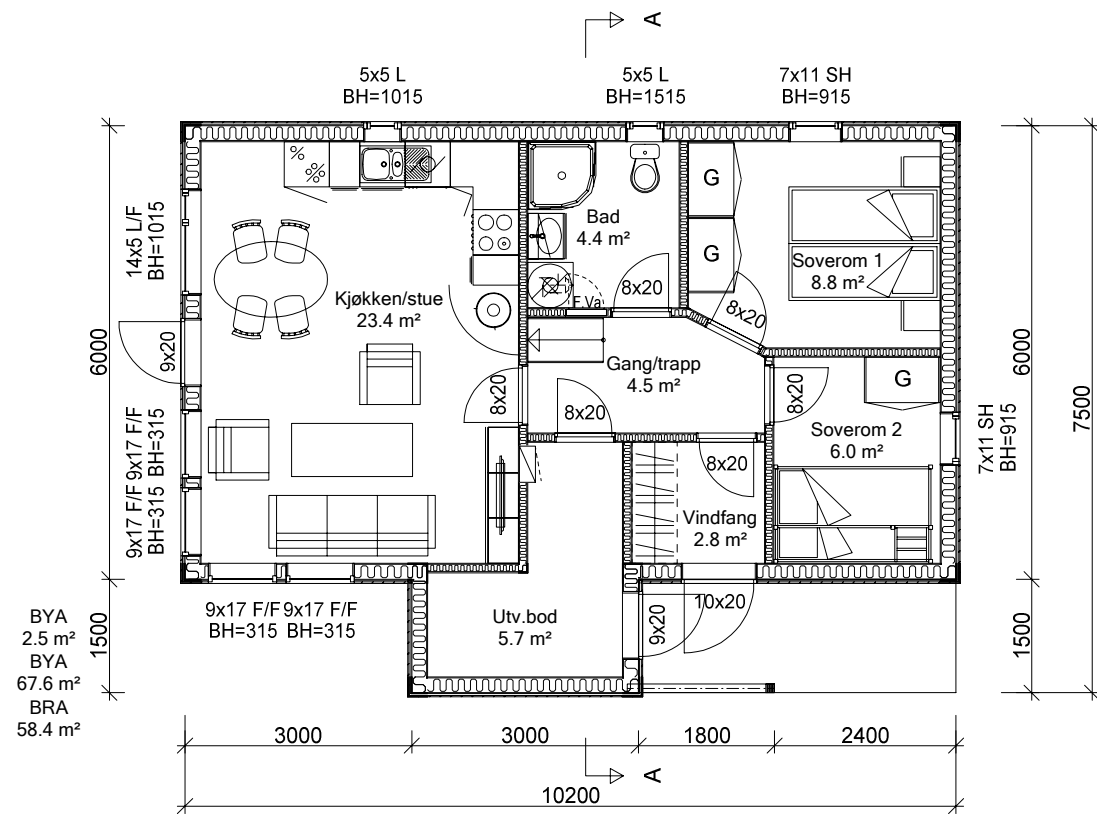
Plan 1. etasje
