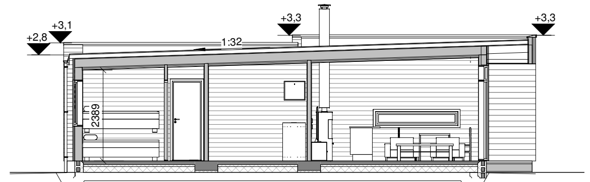
A 1 : 100
