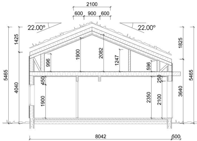
Snitt A-A
