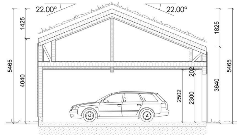
Snitt C-C
