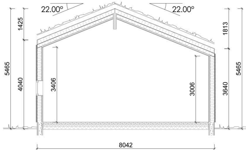
Snitt B-B
