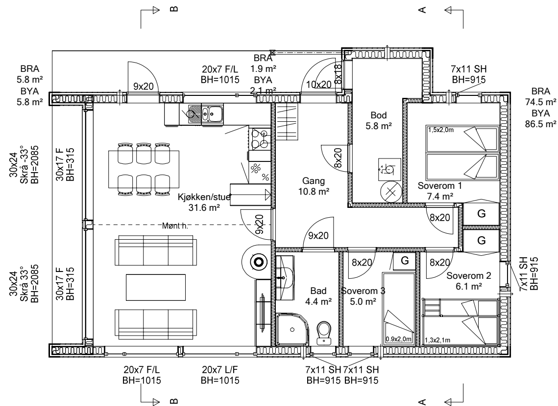
Plan 1. etasje
