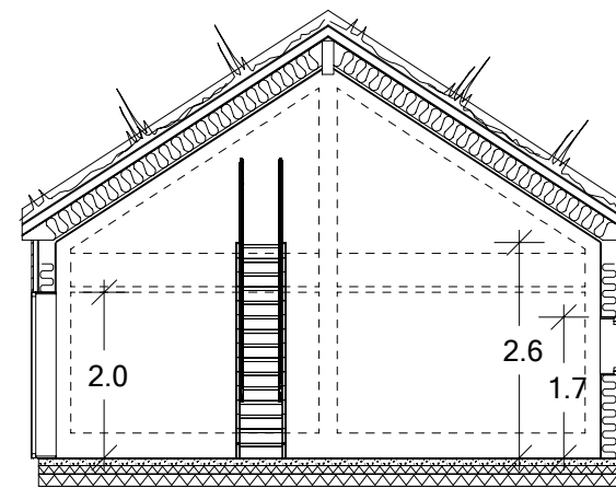
Snitt B-B
