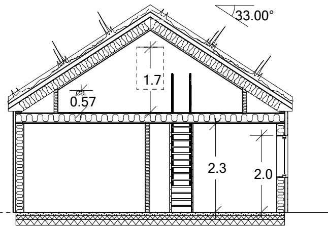
Snitt A-A
