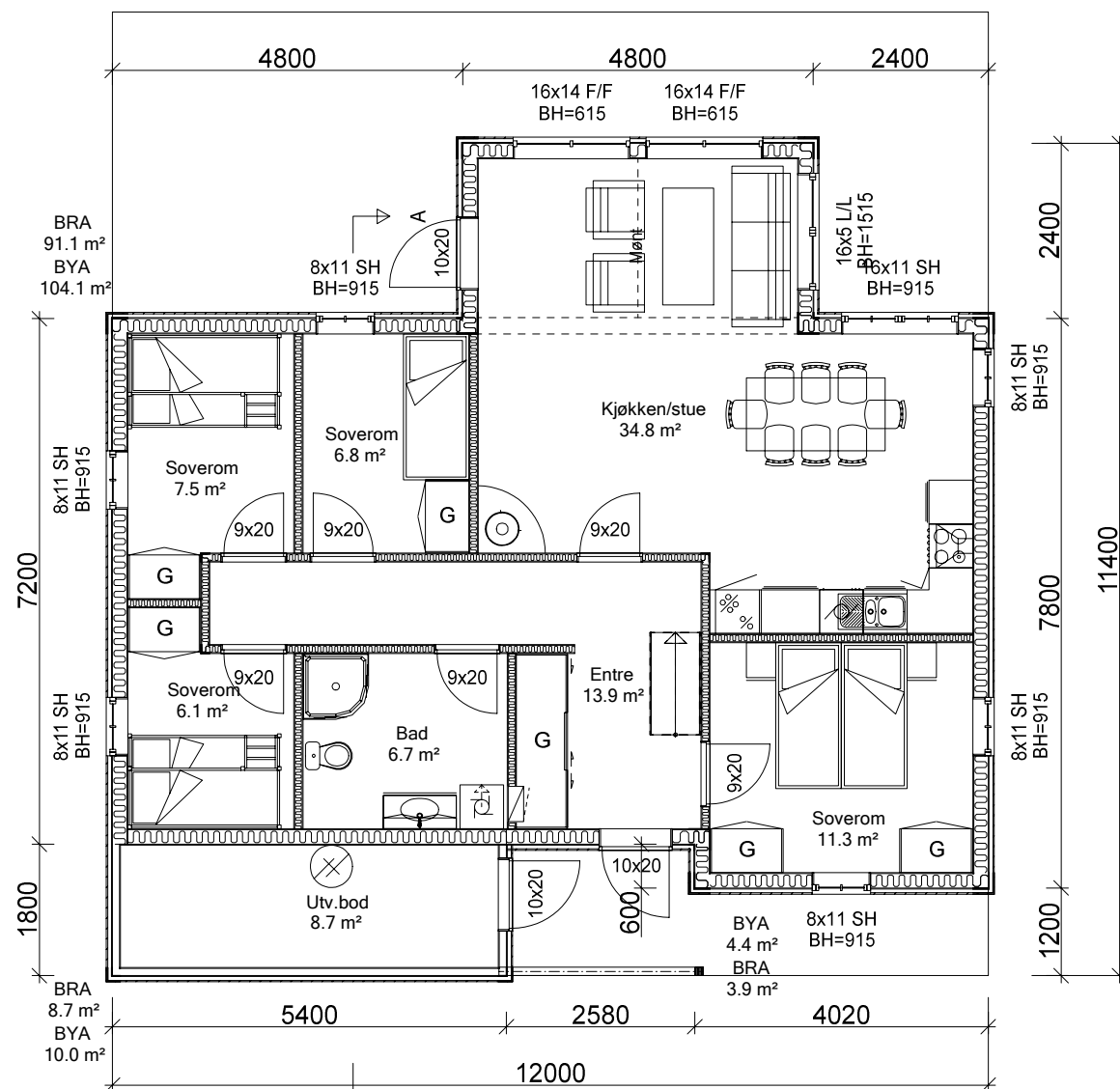
Plan 1. etasje
