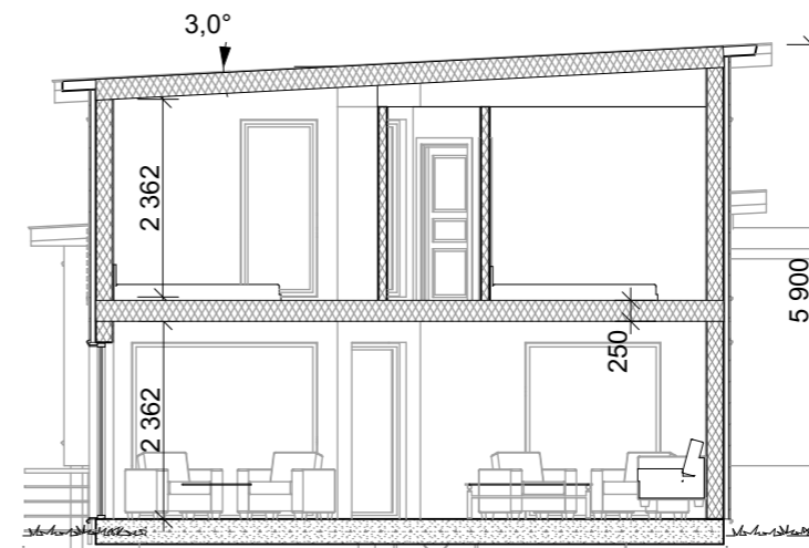
Snitt A-A
