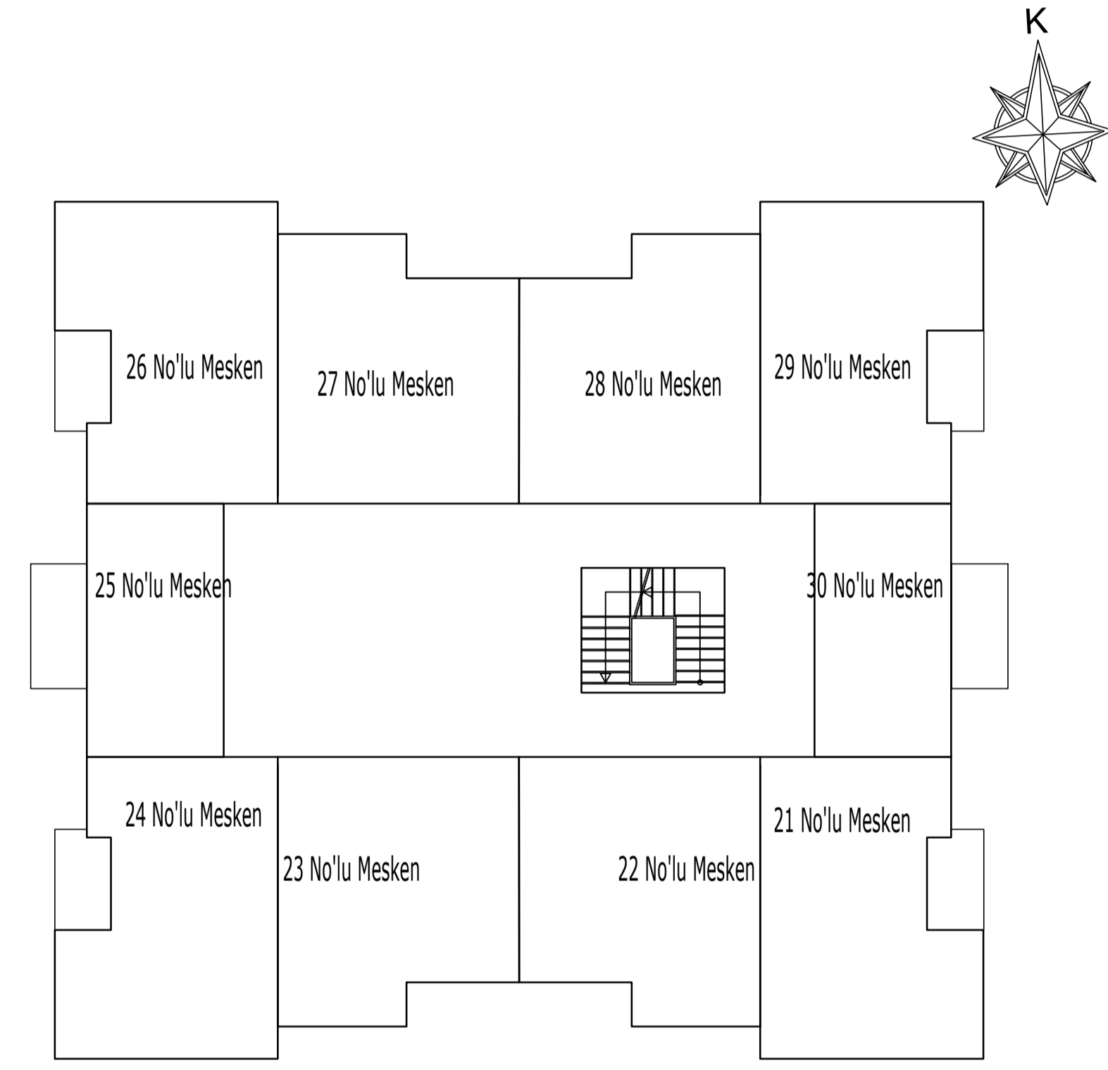
2. KAT
