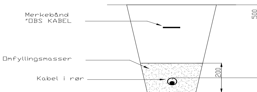
FIG. 1) Krav til kabelgrøft
