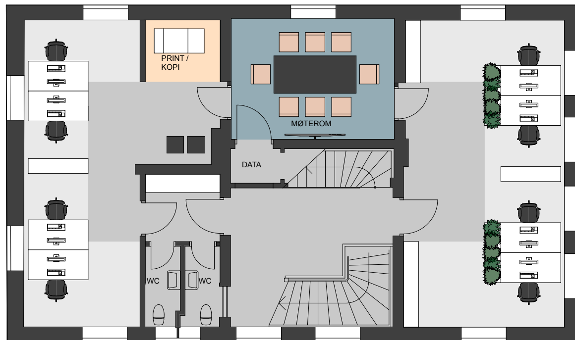
2. ETG - BRA: 118 m2
