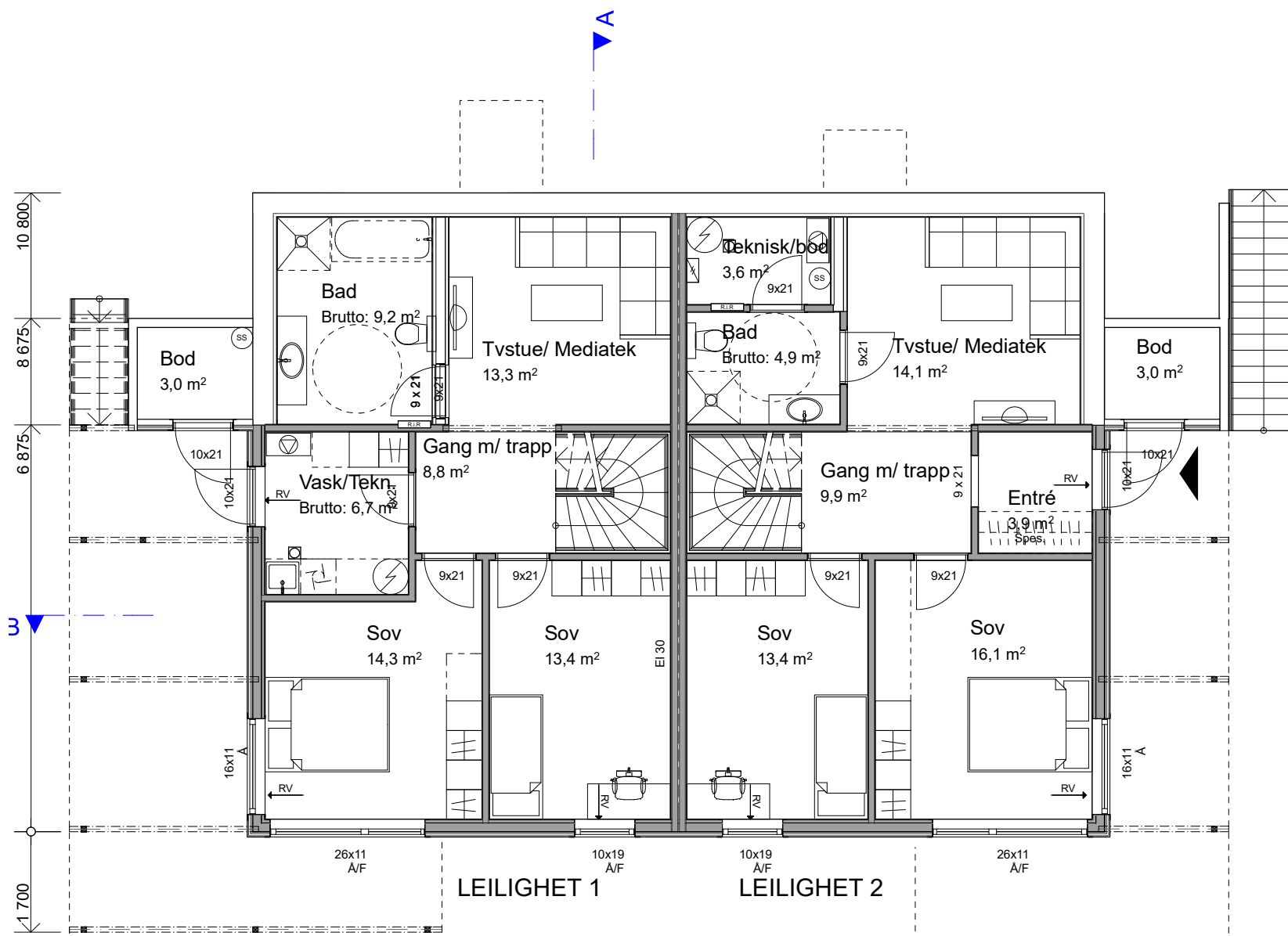
PLAN 1. ETASJE
