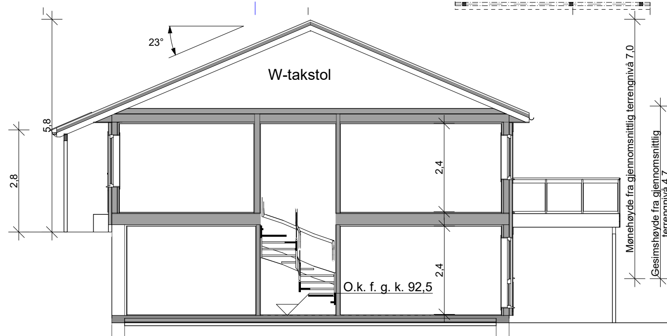
SNITT A-A
