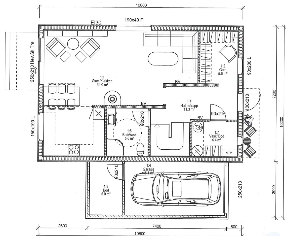
Hovedplan Bya=102,5 m 2 / Bra=91,3 m 2 inkl. garasje
