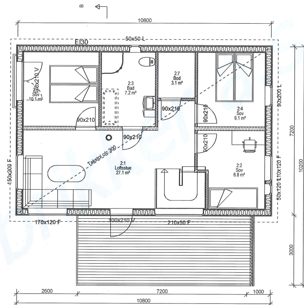
Plan 2. etasje Bra=68,7m 2
