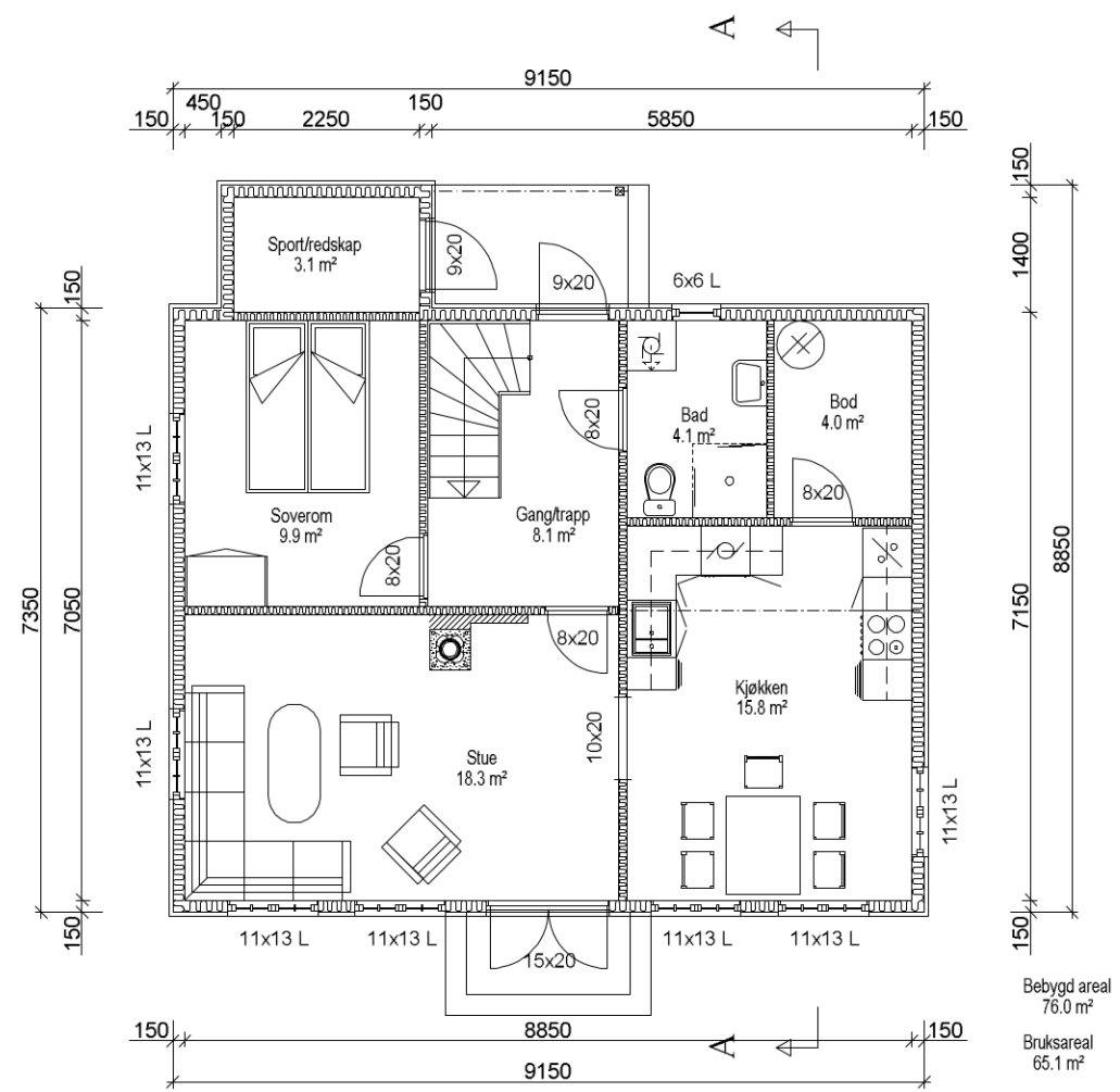
PLAN 1. ETASJE
