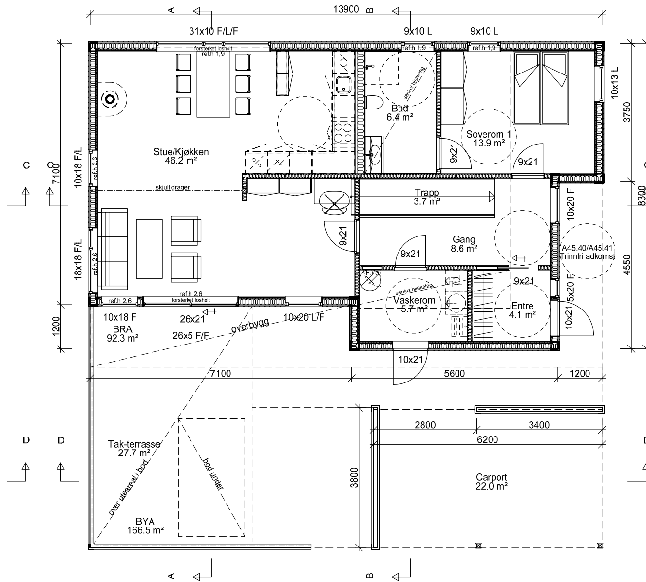
Hovedplan
