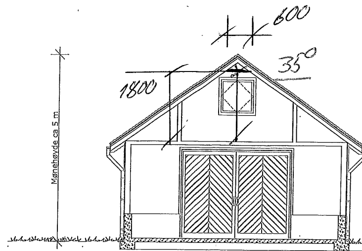
1:100 Snitt A
