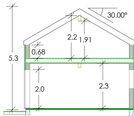
SNITT B - B
