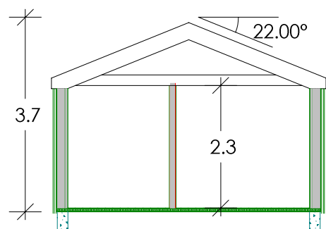
SNITT A - A
