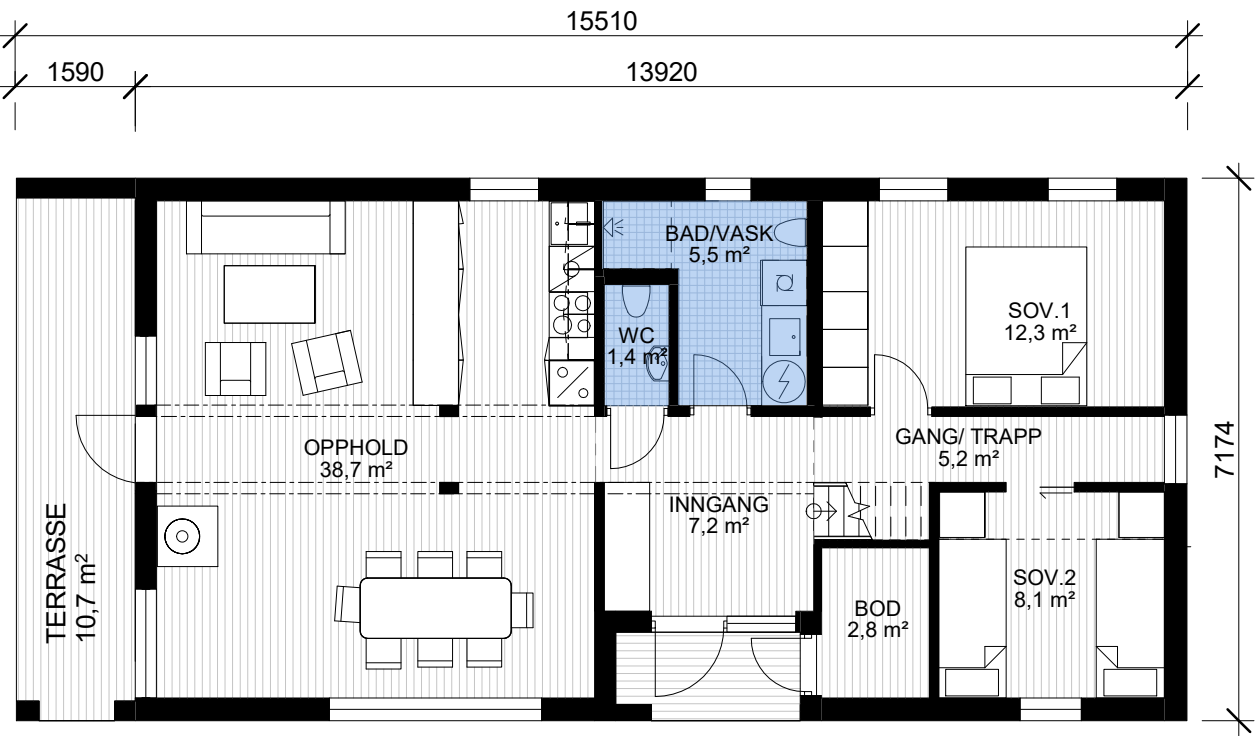
PLAN 1 1 : 100
