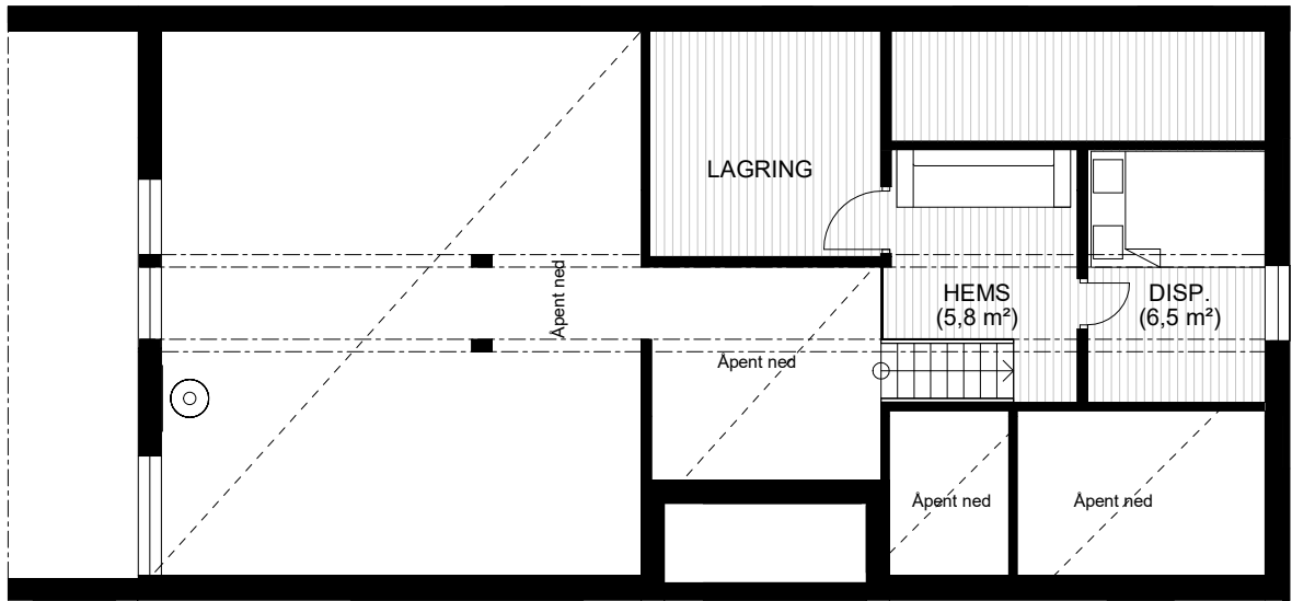
HEMS 1 : 100
