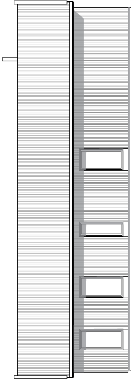
Presentasjon Fasade 3 1 : 100
