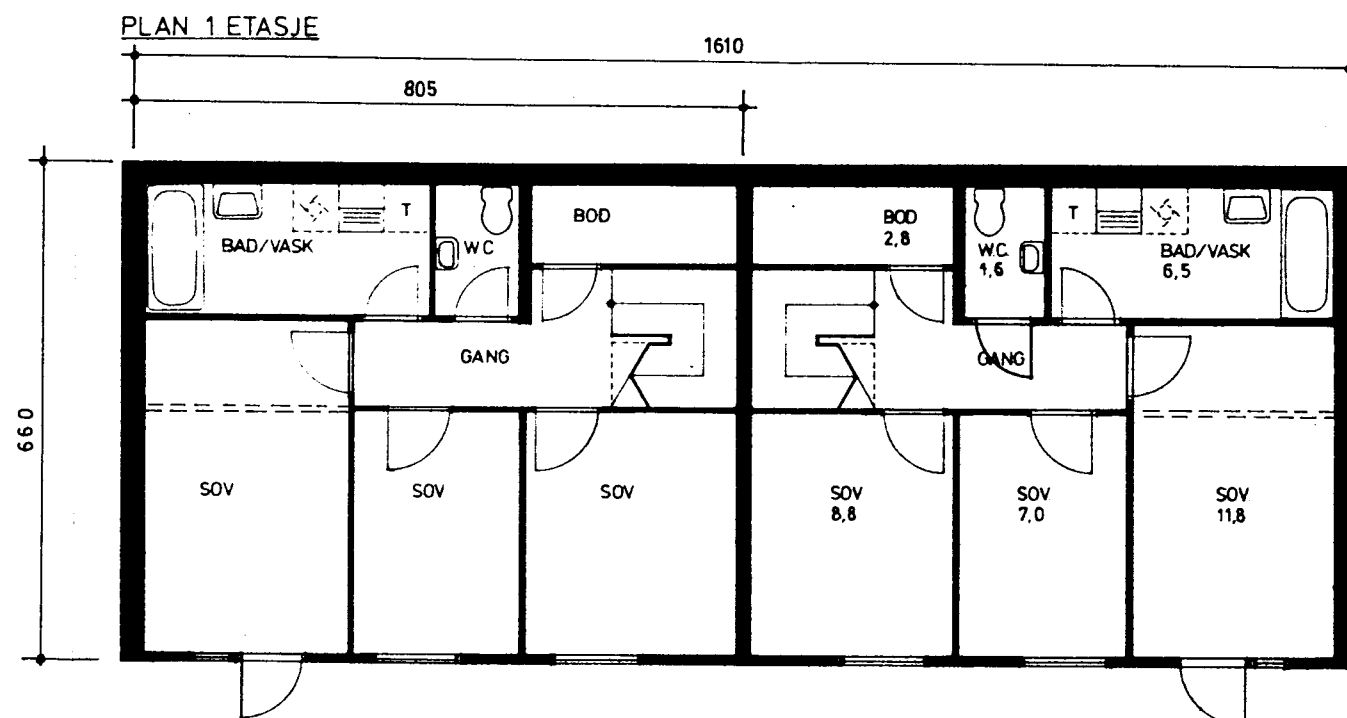
PLAN UNDERETASJE
