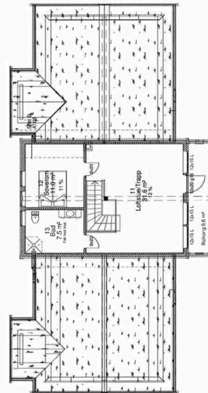
2. Etasje
