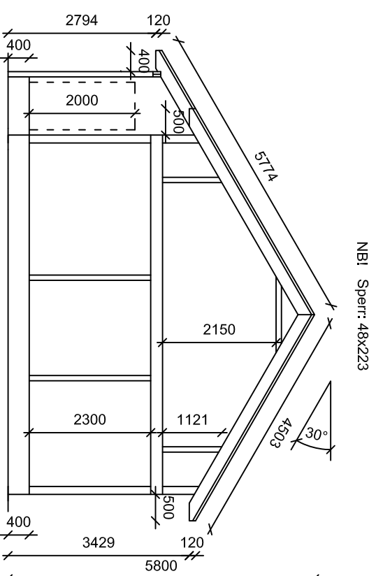
Snitt B - B
