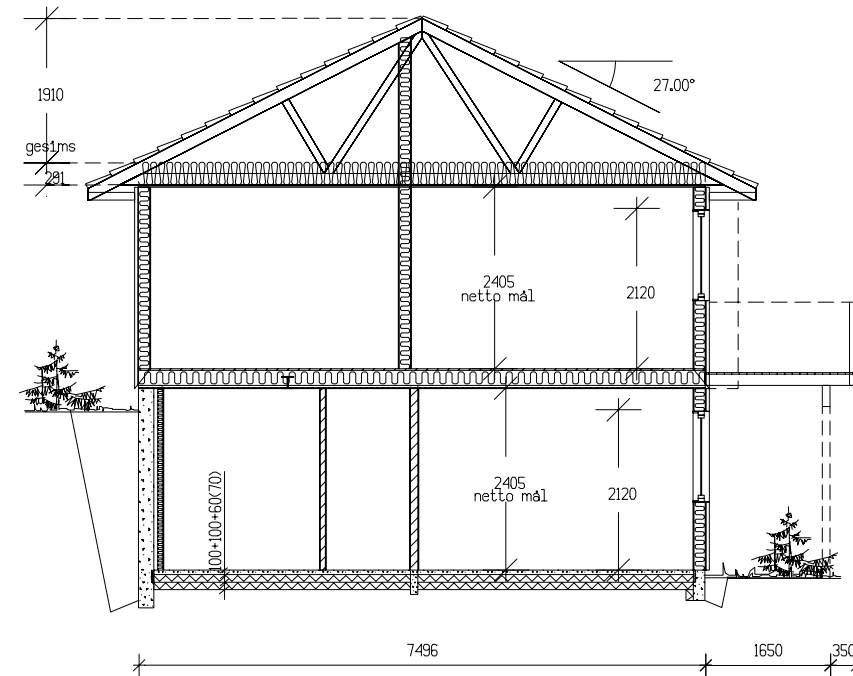
SNITT A-A
